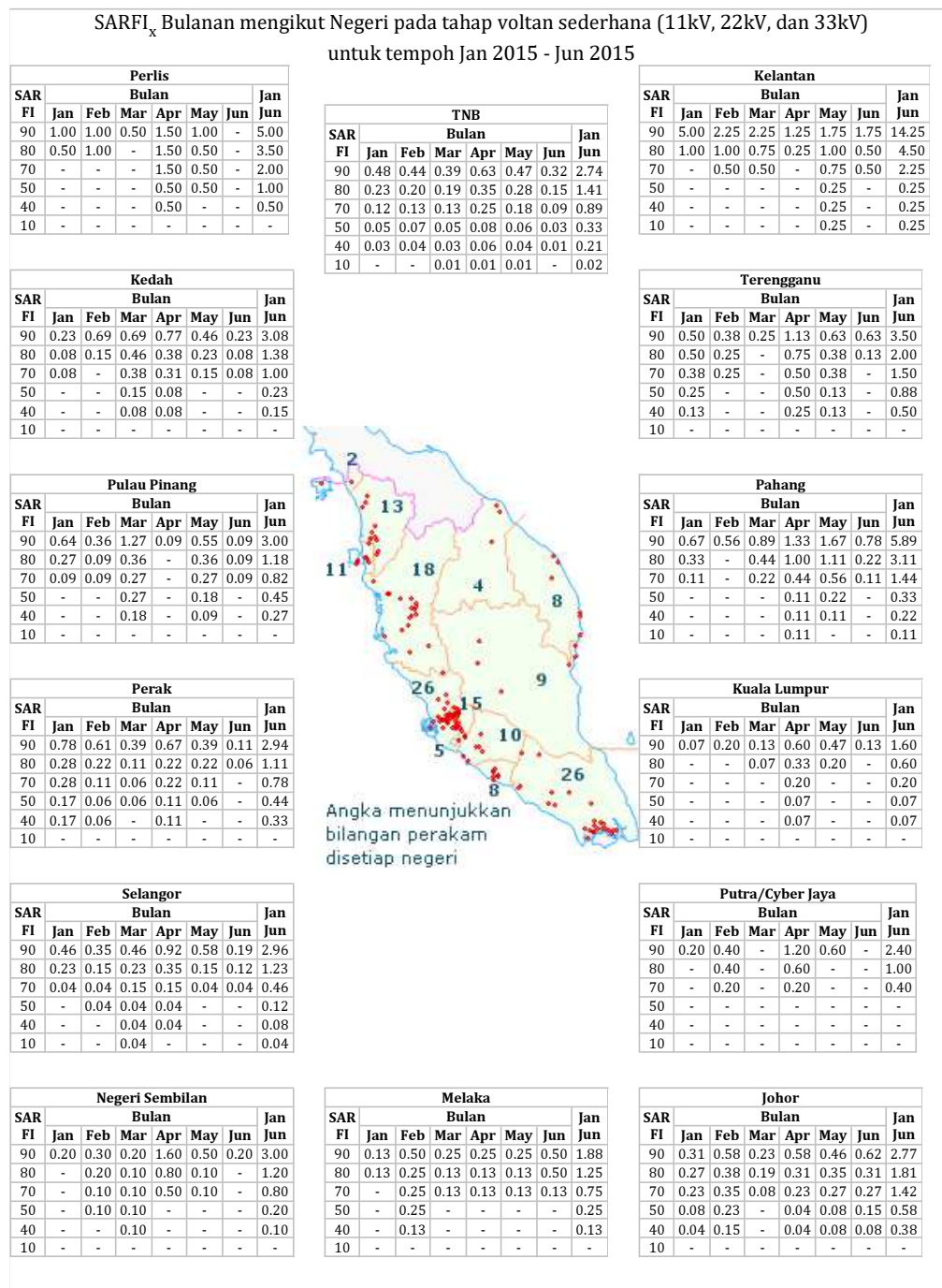
Carta 5: Carta SARFI x mengikut Negeri bagi 1 Januari 2015 hingga 30 Jun 2015
