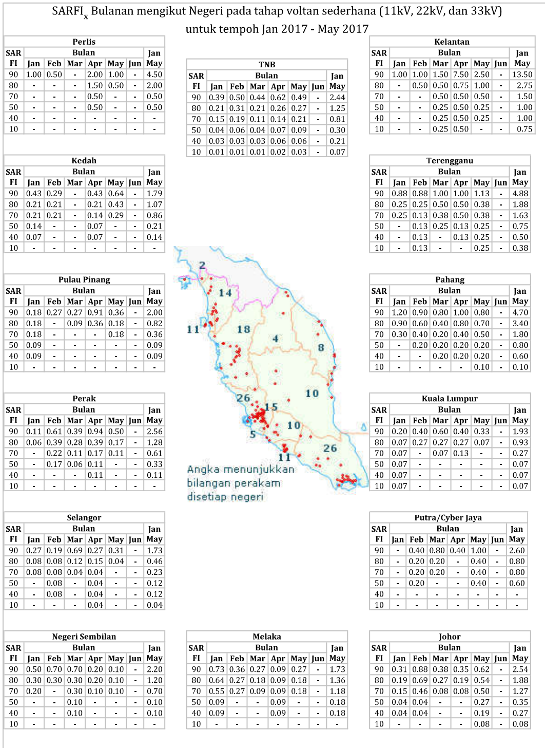
Carta 5: Carta SARFI x mengikut Negeri bagi 1 Januari 2017 hingga 31 Mei 2017
