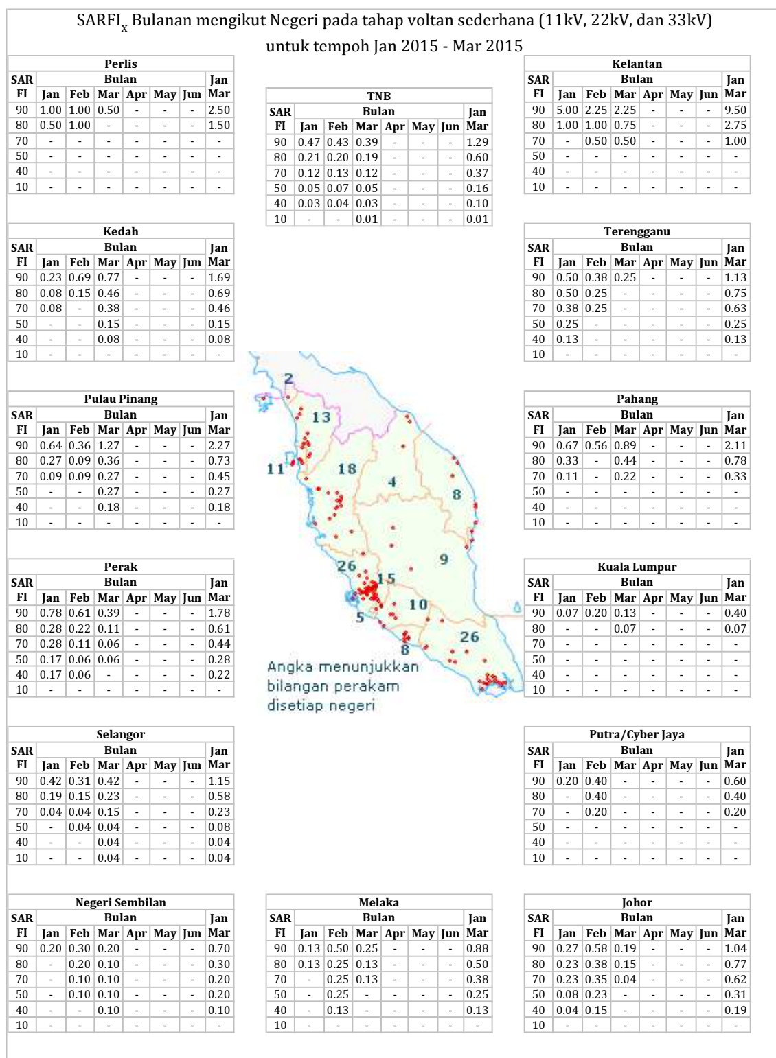
Carta 5: Carta SARFI x mengikut Negeri bagi 1 Januari 2015 hingga 31 Mac 2015
