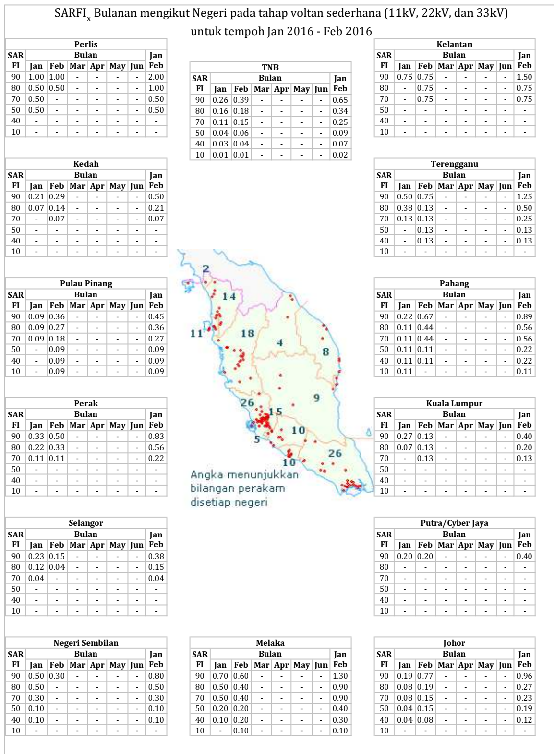
Carta 5: Carta SARFI x mengikut Negeri bagi 1 Januari 2016 hingga 29 Februari 2016
